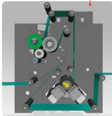
Flexo front - 2 UV
