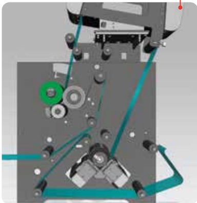
Flexo front - Hot air + UV
