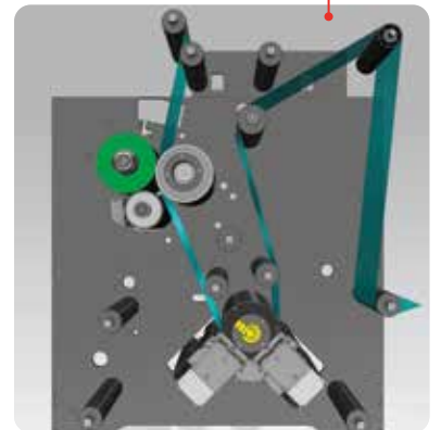
Flexo reverse - 2 UV
